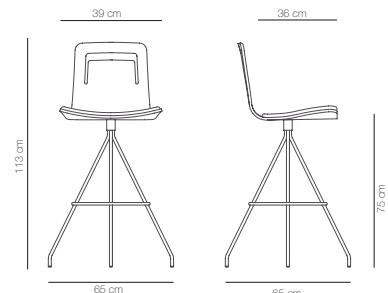
Swivel stool
