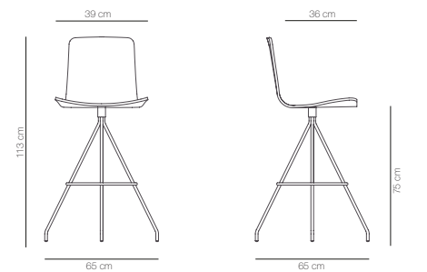
Swivel stool
