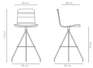
Swivel stool
