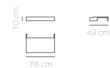
Technical tray Bandeja cubre cableado
